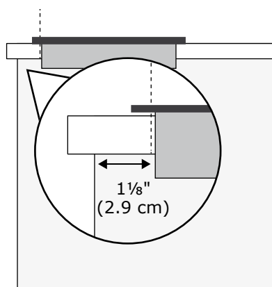
Figure 2b – Distance minimale recommandée depuis l'arrière de l'armoire
