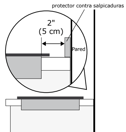
Figura 2c – Distancia mínima recomendada entre el borde posterior del corte y la superficie combustible más cercana detrás de la encimera
