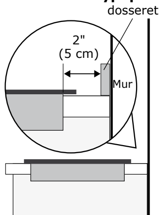
Figure 2c – Distance minimale recommandée entre le bord arrière de la découpe et la surface combustible la plus proche derrière le comptoir
