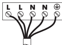
NL 2-phasiger Netzspannungsanschluss
