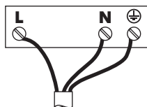
1-phasiger Netzspannungsanschluss
