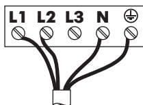
2-phasiger Netzspannungsanschluss
