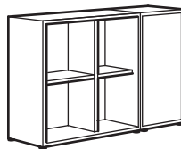
EKET spintelių derinys su kojelėmis. Dydis: P105×G35×A72 cm.
