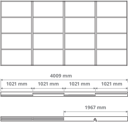
Derinys su ketveriomis durimis ir dvigubu bėgeliu 4 × 1021 mm durys
