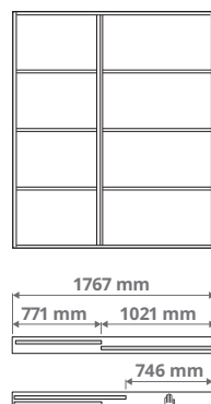
Derinys su dvejomis durimis ir dvigubu bėgeliu 1 × 771 mm ir 1 × 1021 mm durys
