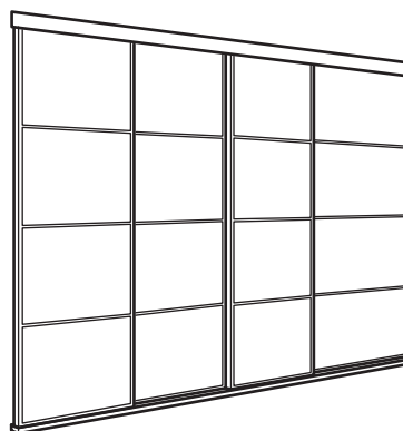
Deriniai su ketveriomis durimis ir dvigubu bėgeliu. 3 x 77 cm ir 1 x 102 cm durys.
