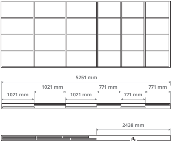
Derinys su šešeriomis durimis ir dvigubu bėgeliu 3 × 771 mm ir 3 × 1021 mm durys
