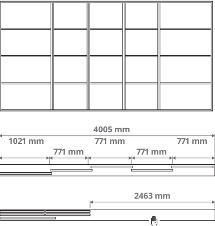
Derinys su penkeriomis durimis ir trigubu bėgeliu 4 × 771 mm ir 1 × 1021 mm durys
