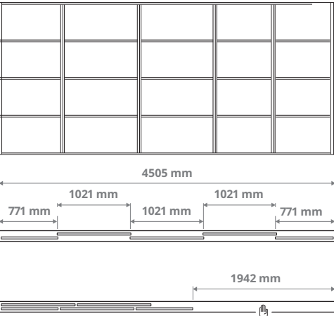
Derinys su penkeriomis durimis ir dvigubu bėgeliu 2 × 771 mm ir 3 × 1021 mm durys
