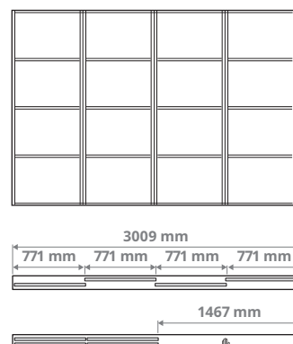
Derinys su ketveriomis durimis ir dvigubu bėgeliu 4 × 771 mm durys
