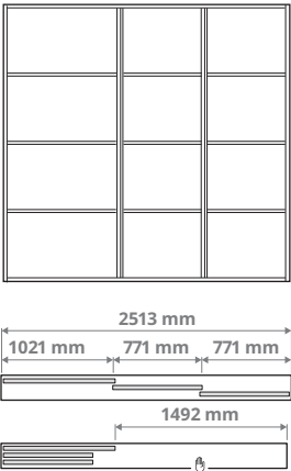
Derinys su trejomis durimis ir trigubu bėgeliu 2 × 771 mm ir 1 × 1021 mm durys
