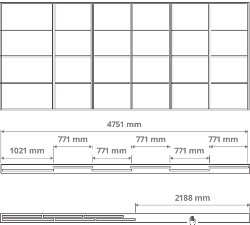
Derinys su šešeriomis durimis ir dvigubu bėgeliu 5 × 771 mm ir 1 × 1021 mm durys
