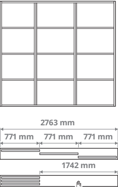
Derinys su trejomis durimis ir trigubu bėgeliu 1 × 771 mm ir 2 × 1021 mm durys
