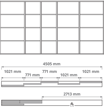
Derinys su penkeriomis durimis ir trigubu bėgeliu 2 × 771 mm ir 3 × 1021 mm durys
