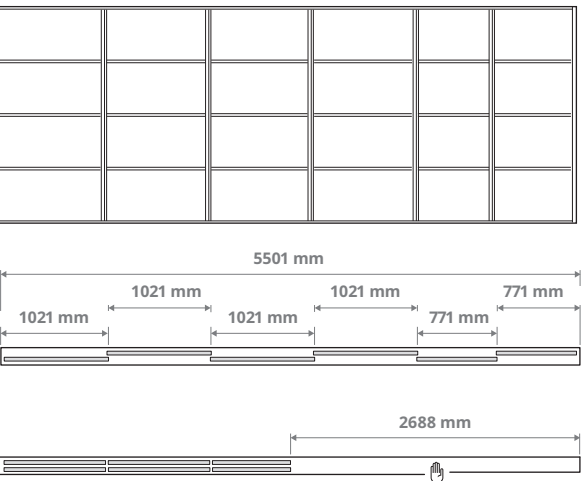
Derinys su šešeriomis durimis ir dvigubu bėgeliu 4 × 1021 mm ir 2 × 771 mm durys
