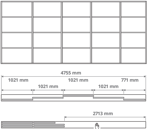
Derinys su penkeriomis durimis ir trigubu bėgeliu 1 × 771 mm ir 4 × 1021 mm durys
