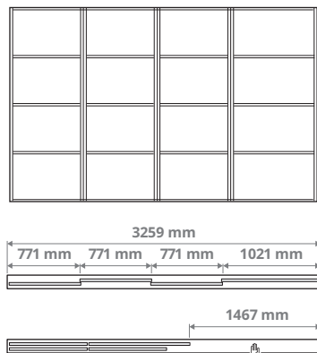
Derinys su ketveriomis durimis ir dvigubu bėgeliu 3 × 771 mm ir 1 × 1021 mm durys
