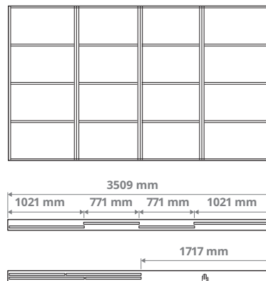
Derinys su ketveriomis durimis ir dvigubu bėgeliu 2 × 771 mm ir 2 × 1021 mm durys
