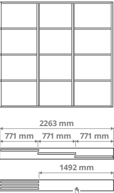
Derinys su trejomis durimis ir trigubu bėgeliu 3 × 771 mm durys
