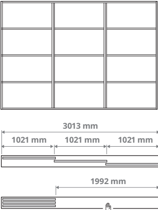
Derinys su trejomis durimis ir trigubu bėgeliu 3 × 1021 mm durys
