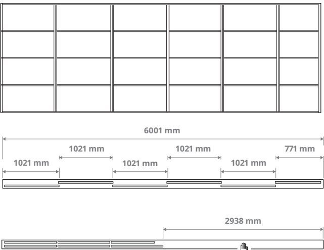
Derinys su šešeriomis durimis ir dvigubu bėgeliu 5 × 1021 mm ir 1 × 771 mm durys
