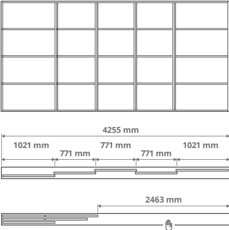
Derinys su penkeriomis durimis ir trigubu bėgeliu 3 × 771 mm ir 2 × 1021 mm durys
