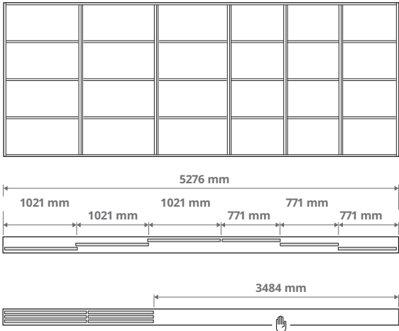
Derinys su šešeriomis durimis ir trigubu bėgeliu 3 × 771 mm ir 3 × 1021 mm durys
