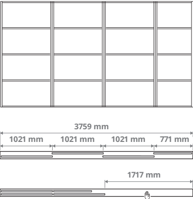
Derinys su ketveriomis durimis ir dvigubu bėgeliu 1 × 771 mm ir 3 × 1021 mm durys
