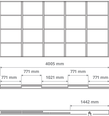
Derinys su penkeriomis durimis ir dvigubu bėgeliu 4 × 771 mm ir 1 × 1021 mm durys
