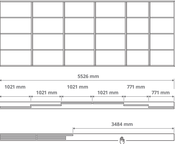
Derinys su šešeriomis durimis ir trigubu bėgeliu 2 × 771 mm ir 4 × 1021 mm durys
