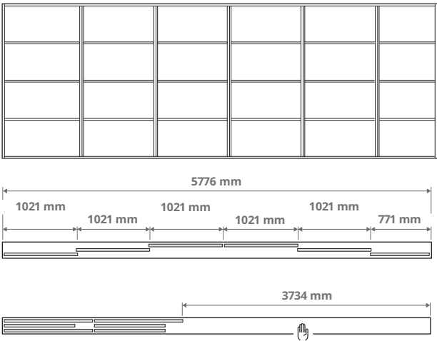
Derinys su šešeriomis durimis ir trigubu bėgeliu 1 × 771 mm ir 5 × 1021 mm durys
