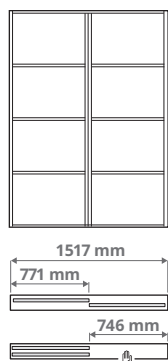
Derinys su dvejomis durimis ir dvigubu bėgeliu 2 × 771 mm durys
