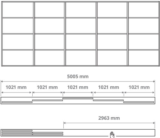
Derinys su penkeriomis durimis ir trigubu bėgeliu 5 × 771 mm
