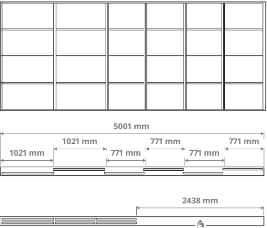
Derinys su šešeriomis durimis ir dvigubu bėgeliu 4 × 771 mm ir 2 × 1021 mm durys
