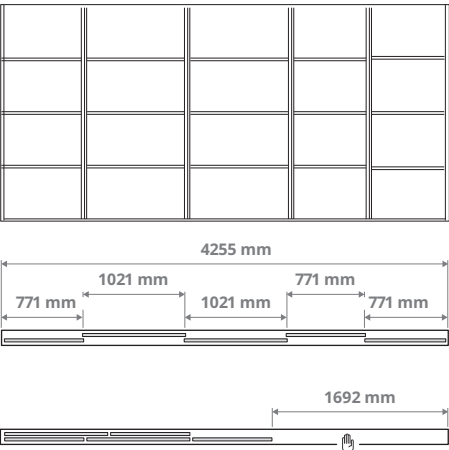
Derinys su penkeriomis durimis ir dvigubu bėgeliu 3 × 771 mm ir 2 × 1021 mm durys
