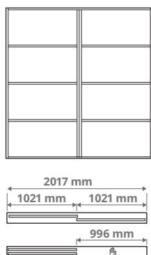
Derinys su dvejomis durimis ir dvigubu bėgeliu 2 × 1021 mm durys
