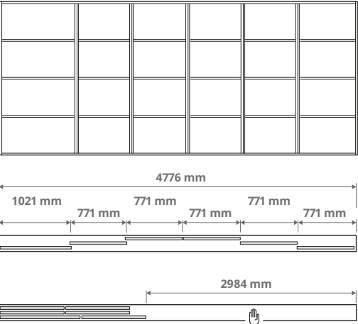
Derinys su šešeriomis durimis ir trigubu bėgeliu 5 × 771 mm ir 1 × 1021 mm durys
