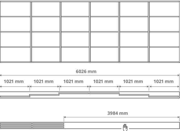
Derinys su šešeriomis durimis ir trigubu bėgeliu 6 × 1021 mm durys
