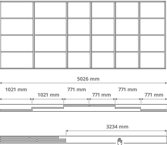
Derinys su šešeriomis durimis ir trigubu bėgeliu 4 × 771 mm ir 2 × 1021 mm durys
