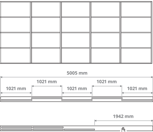
Derinys su penkeriomis durimis ir dvigubu bėgeliu 5 × 1021 mm durys
