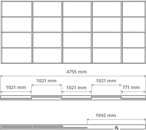
Derinys su penkeriomis durimis ir dvigubu bėgeliu 1 × 771 mm ir 4 × 1021 mm durys
