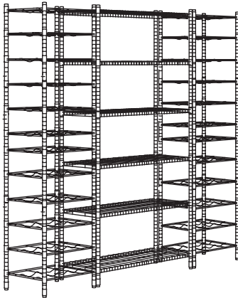
OMAR 오마르 선반유닛 콤비네이션+와인선반, 아연도금. 전체크기: 187×36×181 cm. 콤비네이션 (992.794.80) 쇼핑리스트 OMAR 오마르 와인선반 46×36×94 cm, 아연도금 201.672.11 4개 OMAR 오마르 선반유닛 92×36×94 cm, 아연도금 001.672.07 2개
