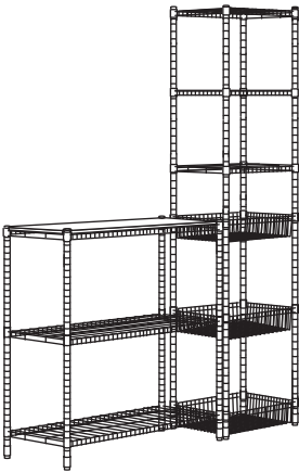
OMAR 오마르 선반유닛 콤비네이션+대나무 선반, 아연도금. 전체크기: 140×36×94~181 cm 콤비네이션 (194.196.96) 쇼핑리스트
