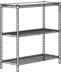
OMAR 오마르 선반유닛/대나무 선반, 그레이그린. 전체크기: 92×36×94 cm 콤비네이션 (694.015.52) 쇼핑리스트
