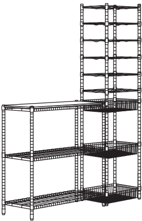
OMAR 오마르 선반유닛 콤비네이션+대나무 선반, 아연도금. 전체크기: 140×36×94~181 cm 콤비네이션 (495.201.60) 쇼핑리스트
