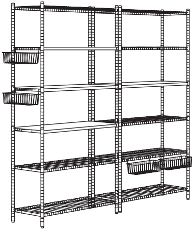
OMAR 오마르 선반유닛 콤비네이션, 아연도금. 전체크기: 197×36×181 cm. 콤비네이션 (692.790.52) 쇼핑리스트 선반유닛 92×36×94 cm, 아연도금 001.672.07 4개 선반커버 92 cm, 아연도금 203.346.63 4개 걸이식바구니, 아연도금 403.346.62 4개
