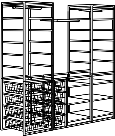
JONAXEL 요낙셀 프레임+철망바구니+조절식옷걸이봉+ 선반유닛 전체 크기: 173×51×173 cm 콤비네이션 (692.976.64)
