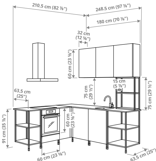
ENHET ר' 210.5 / 248.5 × ע' 63.5 × ג' 226 ס"מ.
