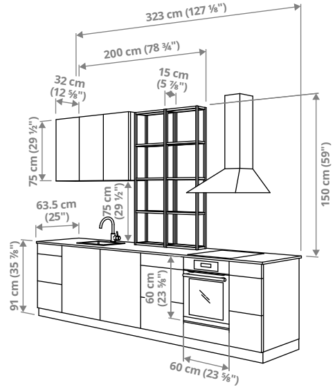
ENHET ר'323 × ע'63.5 × ג'241 ס"מ.
