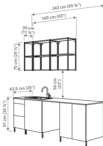
ENHET ר'243 × ע'63.5 × ג'222 ס"מ.
