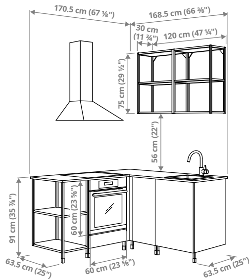
ENHET ר' 170.5 / 168.5 × ע' 63.5 × ג' 222 ס"מ.
