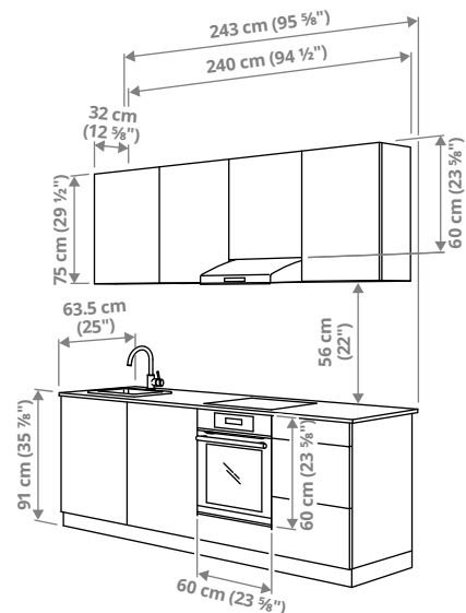
ENHET ר'243 × ע'63.5 × ג'222 ס"מ.
