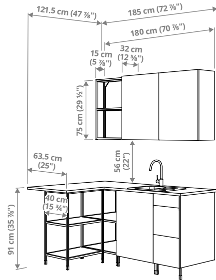
ENHET ר' 121.5 / 185 × ע' 63.5 × ג' 222 ס"מ.
