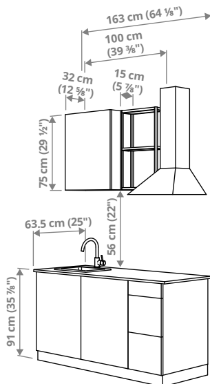
ENHET ר'163 × ע'63.5 × ג'222 ס"מ.
