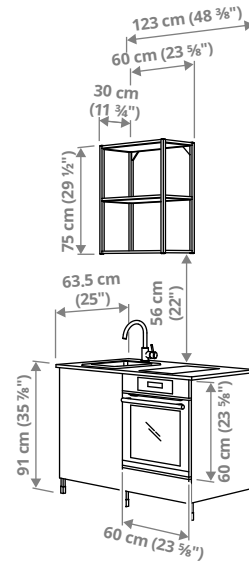
ENHET ר'123 × ע'63.5 × ג'222 ס"מ.
