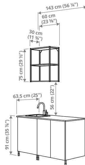
ENHET ר'143 × ע'63.5 × ג'222 ס"מ.
