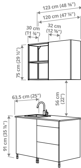
ENHET ר'123 × ע'63.5 × ג'222 ס"מ.
