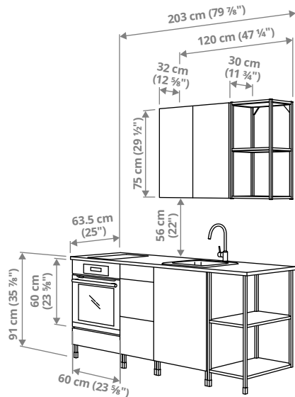
ENHET ר'203 × ע'63.5 × ג'222 ס"מ.
