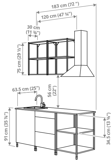
ENHET ר'183 × ע'63.5 × ג'222 ס"מ.
