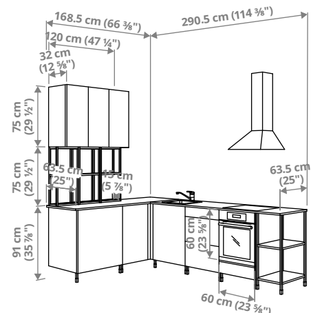
ENHET ר' 168.5 / 290.5 × ע' 63.5 × ג' 241 ס"מ.
