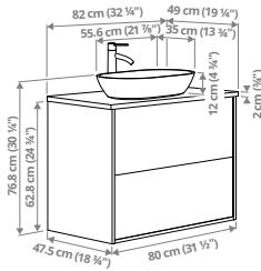
ÄNGSJÖN/OXMYREN ארון תחתון לכיור עם מגירות/כיור/ברד, 82x49x76.8 ס"מ.
