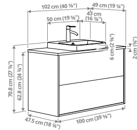
ÄNGSJÖN/BACKSÖN ארון תחתון לכיור עם מגירות/כיור/ברד, 102x49x70.8 ס"מ.
