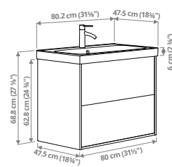
ÄNGSJÖN/BACKSÖN ארון תחתון לכיור עם מגירות/כיור/ברד, 80.2x47.5x68.8 ס"מ.
