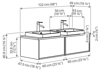
ÄNGSJÖN/BACKSÖN ארון תחתון לכיור עם מגירות/כיורים/ברדים, 122x49x40.8 ס"מ.
