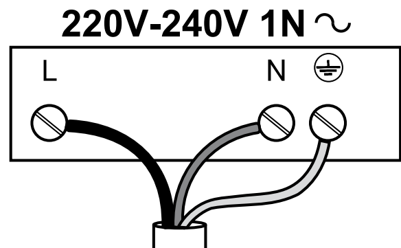
Схема підключення
