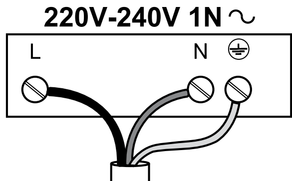
Kytkenäkaavio
