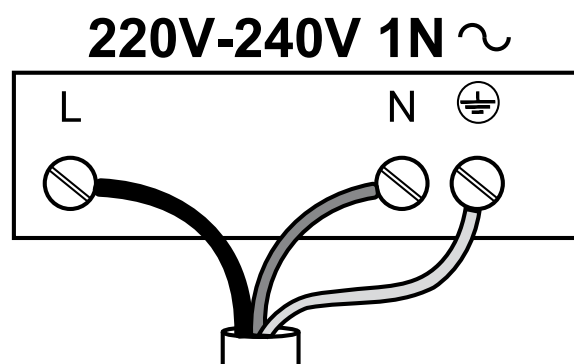
Schemat połączeń
