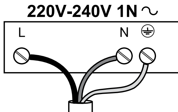
Jungimo schema
