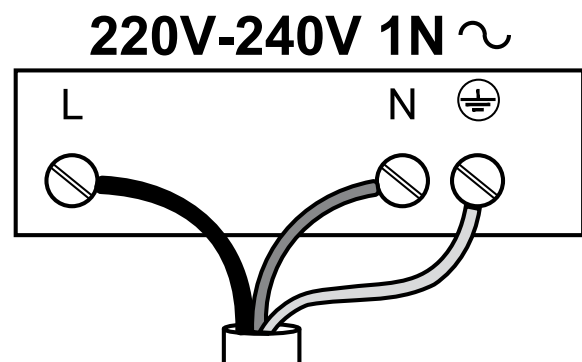
Pieslēguma shēma
