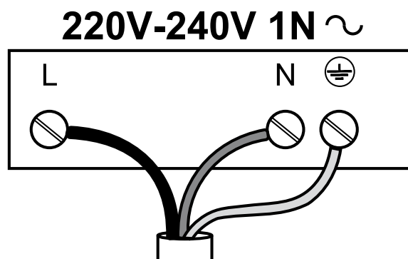
Koblingsskjema
