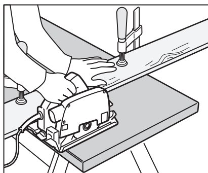
Kui lõikad eelnevalt lõigatud tööpinda, et selle suurst kohandada, kasuta sirge serva säilita-miseks ketassaagi ja pitskruiisid. Kasulik on kasutada ka paari saepukki.
