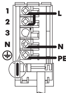
Einphasiger Anschluss 220 V - 240 V ~
