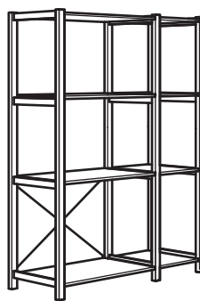
2 secciones/repisas IVAR. Tamaño total: 130×50×179 cm. Pino (492.483.25)
