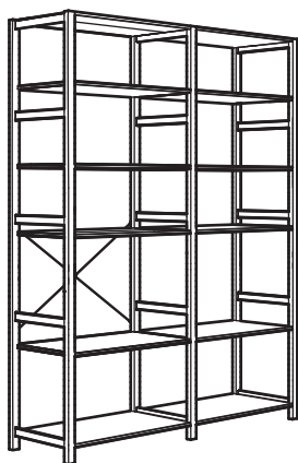
2 secciones/repisas IVAR. Tamaño total: 174×50×226 cm. Pino (492.483.54)
