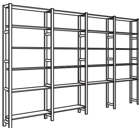
4 secciones/repisas IVAR. Tamaño total: 344×226 cm. Pino (092.485.44)
