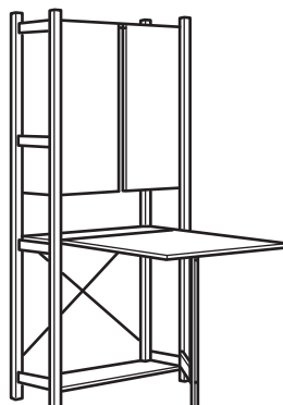
1 sección/estante con mesa plegable IVAR. Tamaño total: 89×30×179 cm. Pino (894.232.23)
