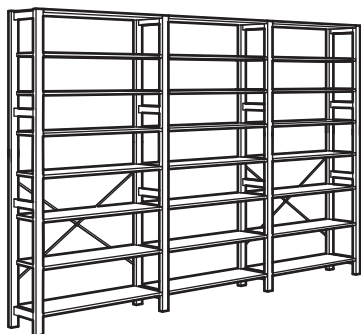
3 secciones/repisas IVAR. Tamaño total: 259×30×179 cm. Pino (692.483.86)
