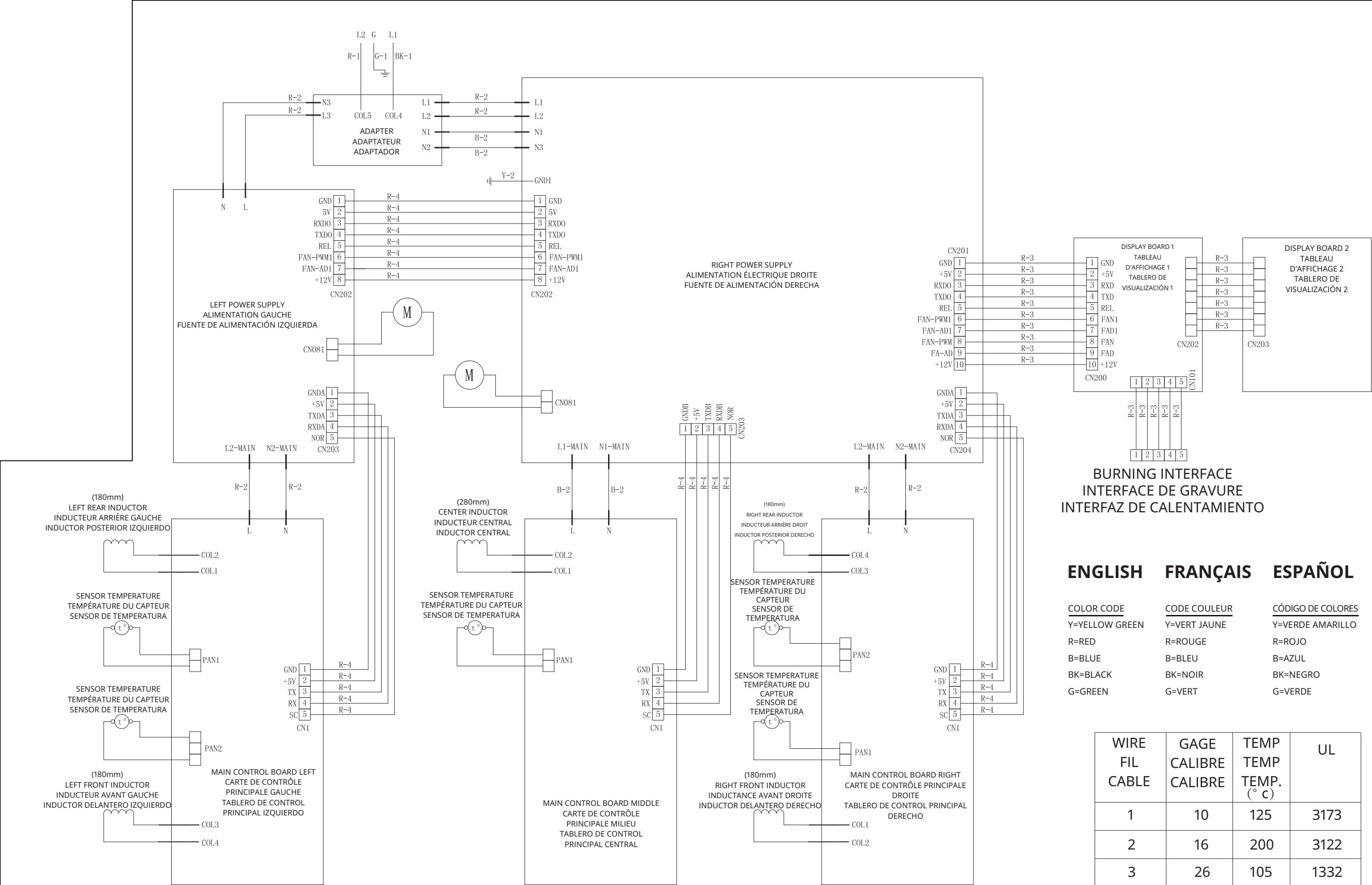
NEDERSTA SCHEMATIC DIAGRAM NEDERSTA SCHÉMA GRAPHIQUE NEDERSTA DIAGRAMA ESQUEMÁTICO
