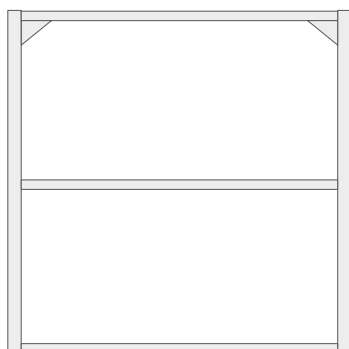
Étagère inférieure 24po (H60,9cm) Dimensions: 18×18po (L45,7×P45,7cm)
