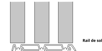
Vue latérale d'un rail à trois voies avec portes
