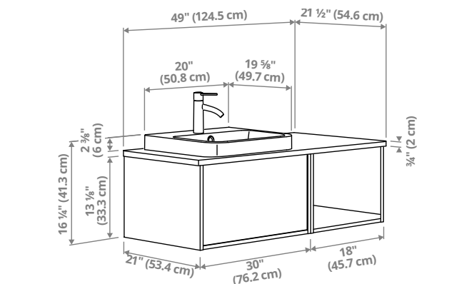
ÄNGSJÖN/BACKSJÖN. Meuble pour lavabo à tiroir, lavabo et mitigeur. 124,5×54,6×41,3cm (49×21½×16¼po)
