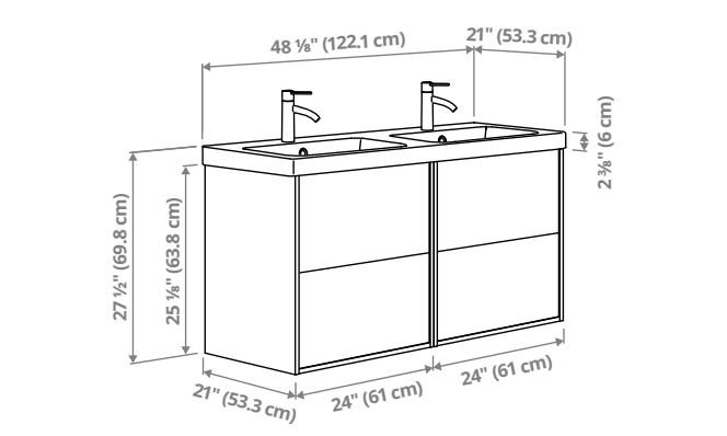
ÄNGSJÖN/BACKSJÖN. Meuble pour lavabo à tiroirs, lavabo et mitigeurs. 122,1×53,3×69,8cm (48⅛×21×27½po)
