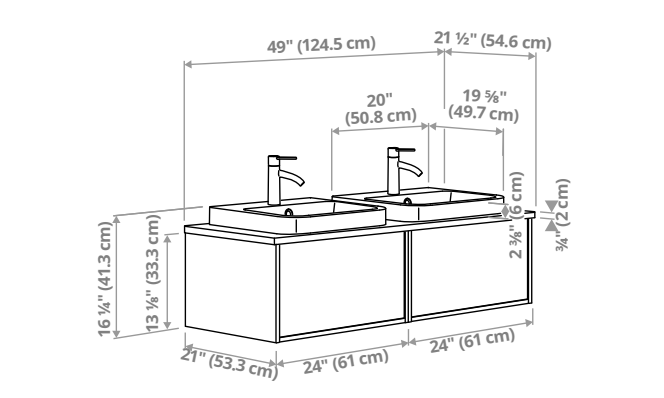
ÄNGSJÖN/BACKSJÖN. Meuble pour lavabo à tiroirs, lavabos et mitigeur. 124,5×54,6×41,3cm (49×21½×16¼po)
