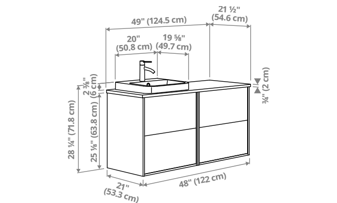
ÄNGSJÖN/BACKSJÖN. Meuble pour lavabo à tiroirs, lavabo et mitigeur. 124,5×54,6×71,8cm (49×21½×28¼po)
