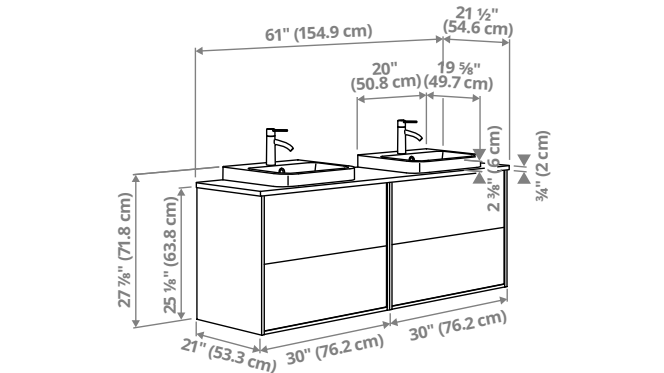
ÄNGSJÖN/BACKSJÖN. Meuble pour lavabo à tiroirs, lavabos et mitigeurs. 154,9×54,6×71,8cm (61×21½×28¼po)
