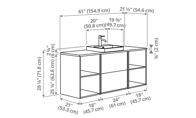
ÄNGSJÖN/BACKSJÖN. Meuble pour lavabo à tiroirs, lavabo et mitigeur. 154,9×54,6×71,8cm (61×21½×28¼po)
