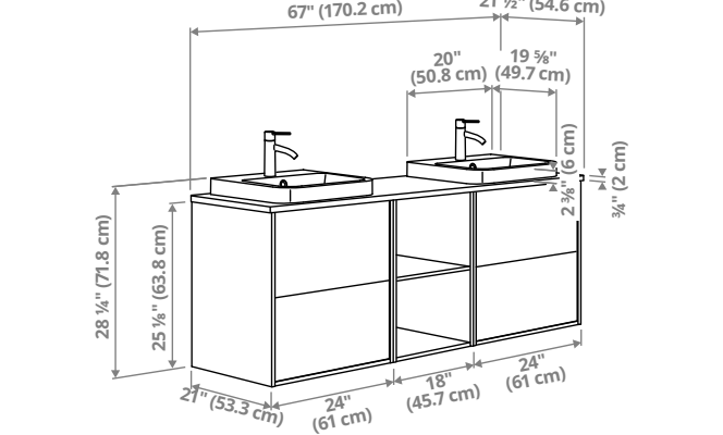
ÄNGSJÖN/BACKSJÖN. Meuble pour lavabo à tiroirs, lavabos et mitigeurs. 170,2×54,6×71,8cm (67×21½×28¼po)
