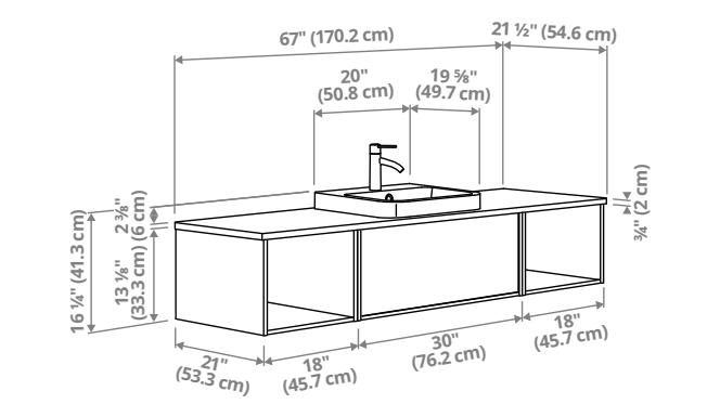
ÄNGSJÖN/BACKSJÖN. Meuble pour lavabo à tiroir, lavabo et mitigeur. 170,2×54,6×41,3cm (67×21½×16¼po)
