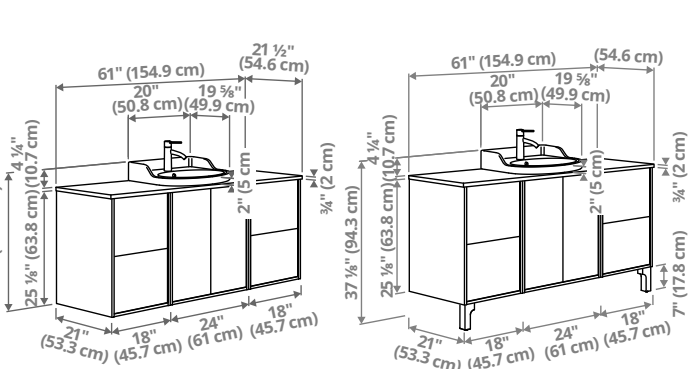
TÄNNFORSEN/RUTSJÖN. Meuble pour lavabo à portes et à tiroirs, lavabo, et mitigeur. 154,9×54,6×76,5cm (61×21½×30⅛po) sans pieds
