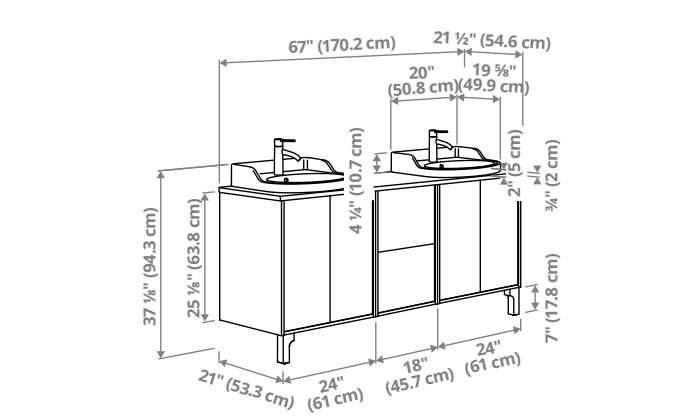
TÄNNFORSEN/RUTSJÖN. Meuble pour lavabo à tiroirs et à portes, lavabos et mitigeurs. 170,2×54,6×94,3cm (67×21½×37⅞po)
