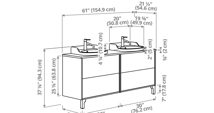
TÄNNFORSEN/RUTSJÖN. Meuble pour lavabo à tiroirs, lavabos et mitigeurs. 154,9×54,6×94,3cm (61×21½×37⅞po)
