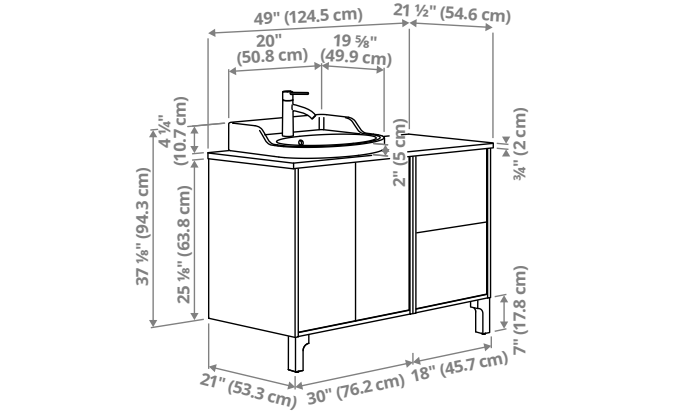
TÄNNFORSEN/RUTSJÖN. Meuble pour lavabo à portes et tiroirs, lavabo et mitigeur. 124,5×54,6×94,3cm (49×21½×37⅞po)
