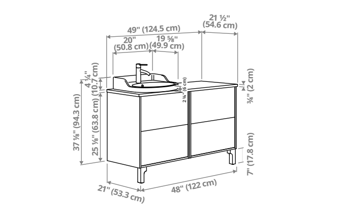
TÄNNFORSEN/RUTSJÖN. Meuble pour lavabo, lavabo et mitigeur. 124,5×54,6×94,3cm (49×21½×37⅞po)
