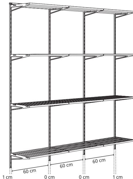
Example 2: 1\text{ cm} + 60\text{ cm} + 60\text{ cm} + 60\text{ cm} + 1\text{ cm} = 182\text{ cm}
