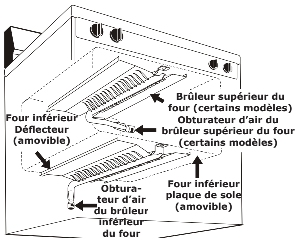
Fig. 19 - Emplacement des brûleurs du four
