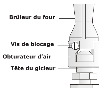
Fig. 20 - Obturateur d'air du brûleur du four
