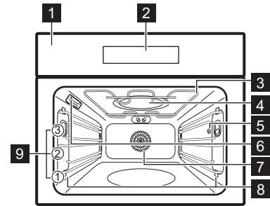
1 Käyttöpaneeli
