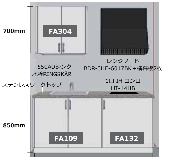
呼び寸法 1400mm 奥行650mm (カバーパネル含み実寸 1422~1430mm 面材による)
